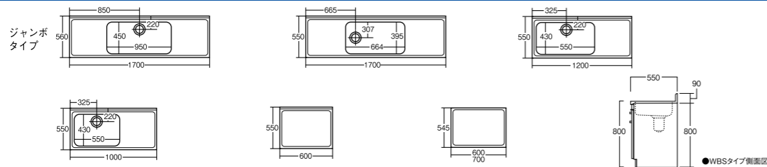
ガス台 二段引出し付 バックガード付 WBS-70GBF ¥82,800 (税別) 寸法:間口700×奥行545×高さ610+280
